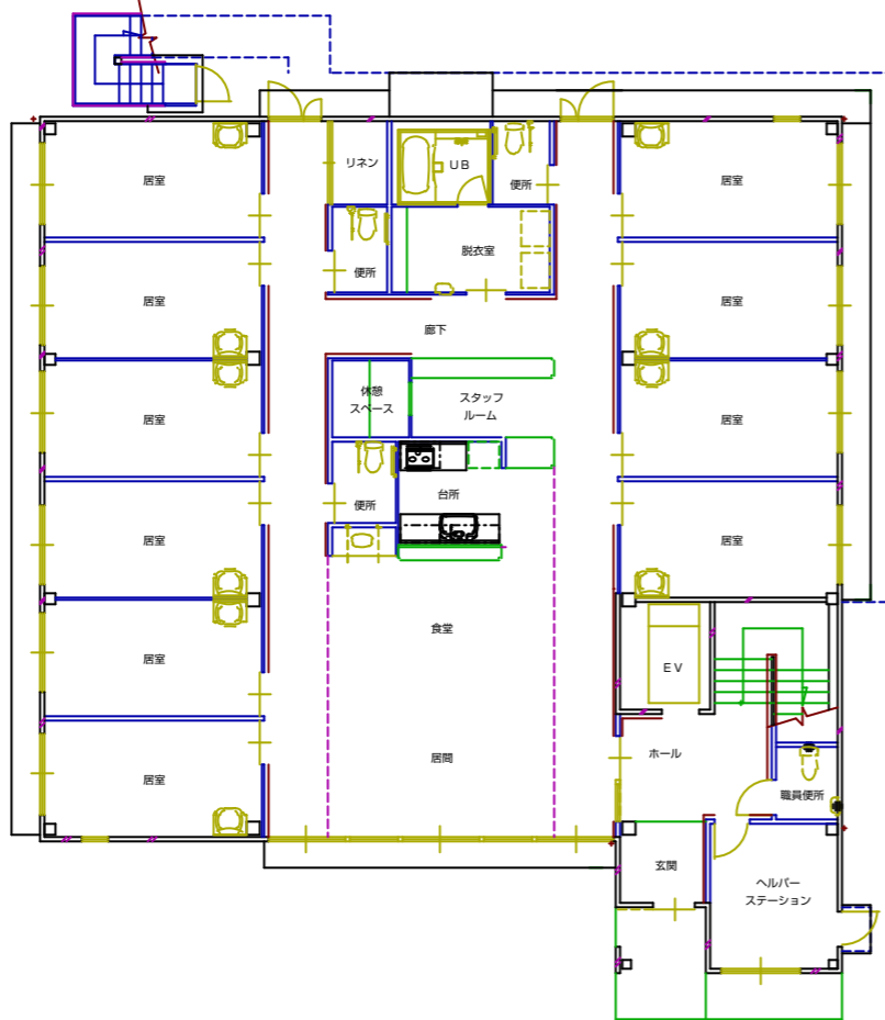
1階平面図 1:100
