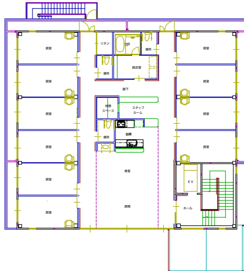
2階平面図 1:100
